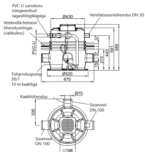
Sinkamat-K (Tootekoodid 620387, 620490)
