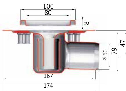
Standardne renn
