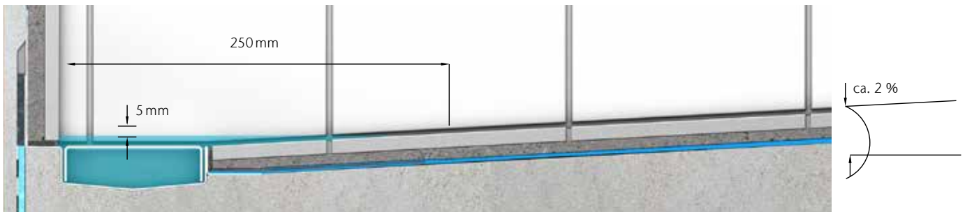
Veesammas seinääärsse paigalduse puhul
