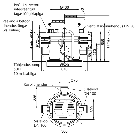
Sinkamat-K (Tootekoodid 620441, 620491)
