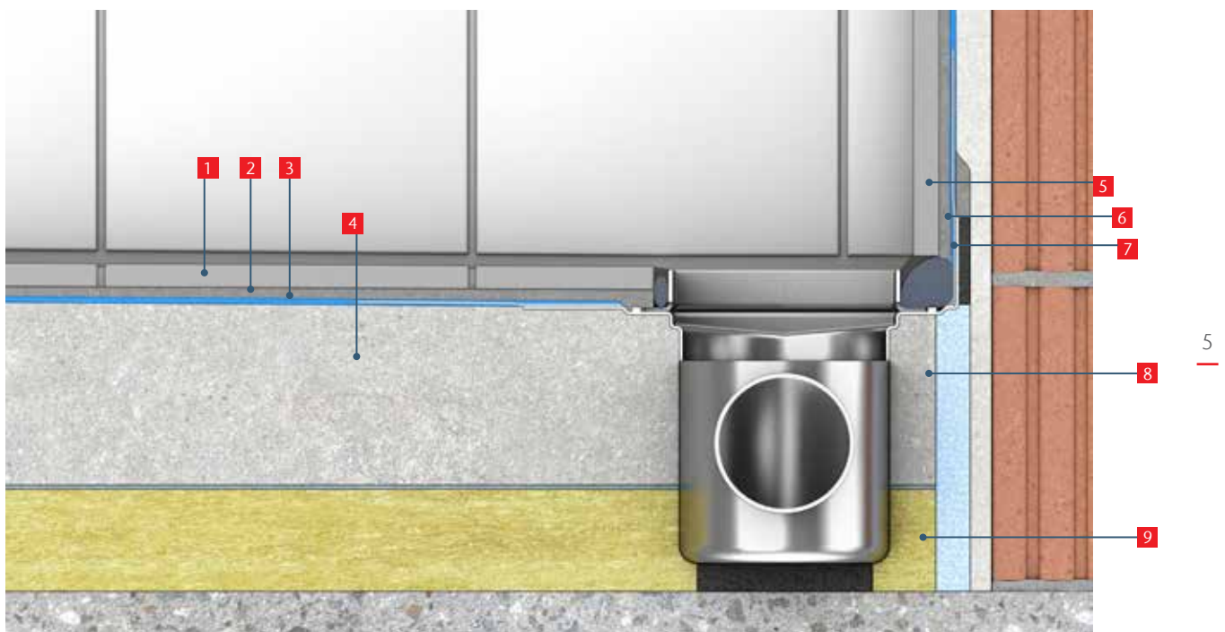
Soovitav paigaldamine ShowerDrain E+ näitel
