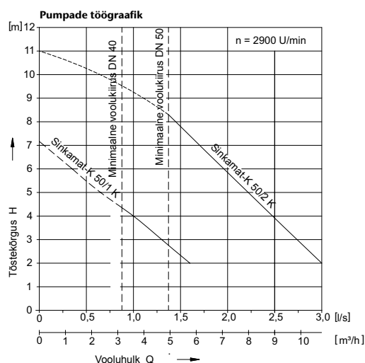
Sinkamat-K (Tootekoodid 620442, 620492)
