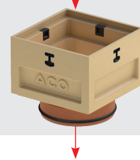
Ülaosa ümara trapi jaoks, DN 200 toote nr. 319602
