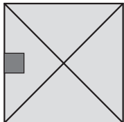
Keraamiline plaat min 640x640 mm
