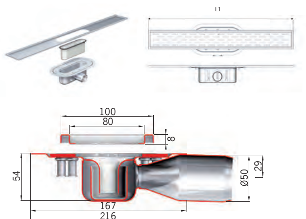
Madal renn
