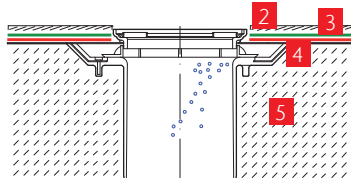
Dušitrapp nõrgumisvõimalusega
