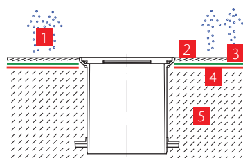
Dušitrapp nõrgumisvõimalusega
