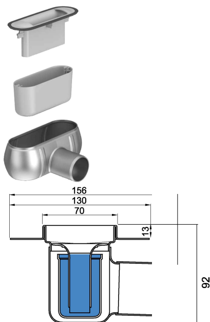
Standardne renn (kogukõrgus 92 mm)
