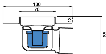
Madal renn (kogukõrgus 65 mm)
